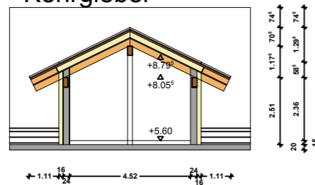
Querschnitt Kehrgiebel
